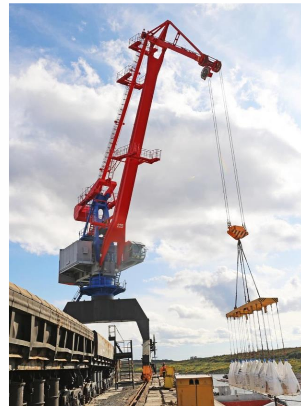
Кран порталный «Зубр» КПП 16(20/32)-32/25-10,5К
