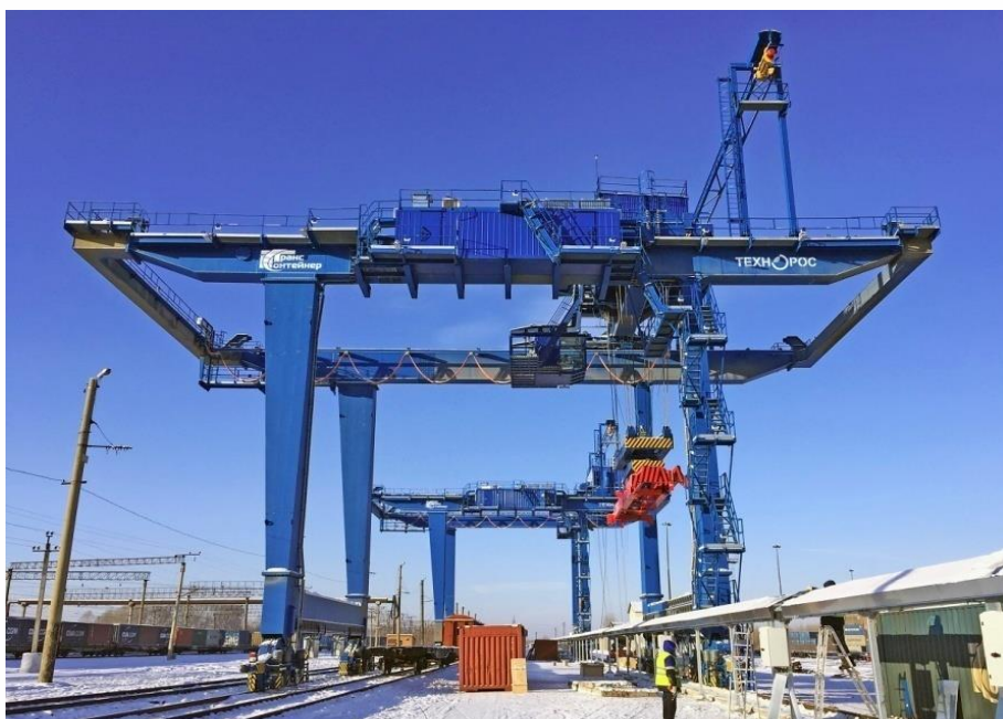
Краны козловые контейнерные КК-Кнт 45-16/4,5/6-12,5, А6,У1
